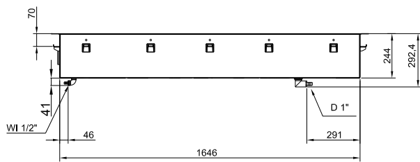
Sivulta
